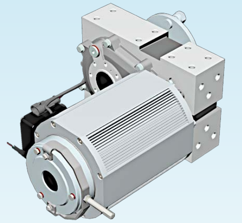
DD1 SERIE WHEEL DRIVE
