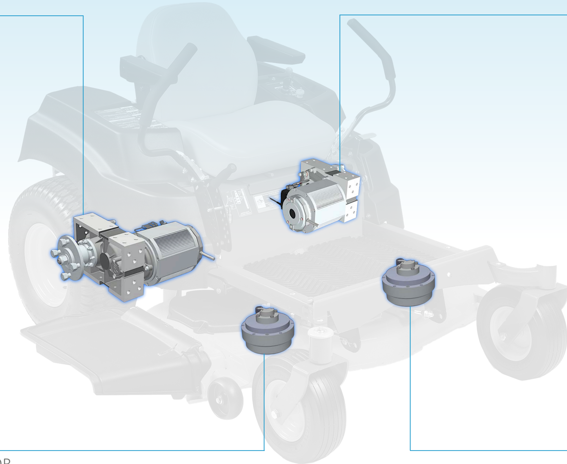
DD1 SERIE WHEEL DRIVE
